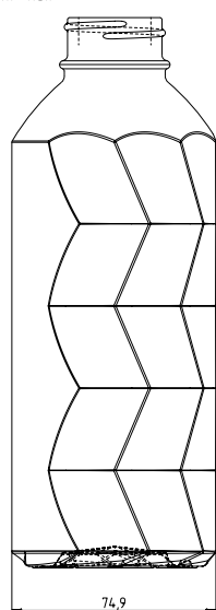
Pogled od spredaj Front view
