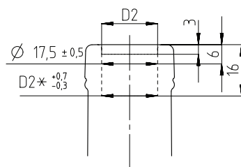
Profil luknje Hole profile
